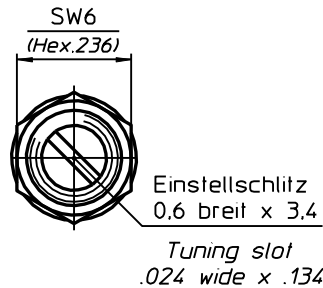
Einbaumaß Mounting layout
