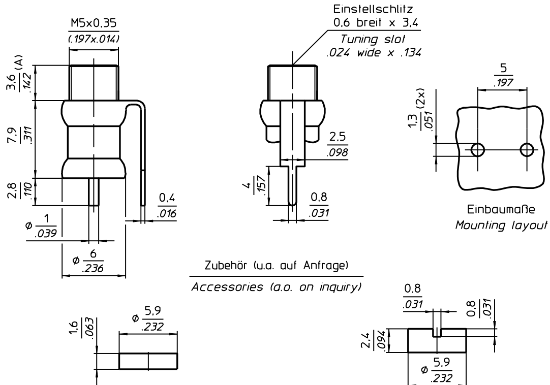
Dichtkappe : Maß A+0,5 Seal cap : Dim A+.02
