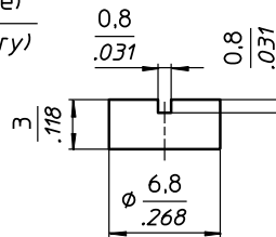
Dichtkappe geschlitzt : Maß A+1,4 Slotted seal cap : Dim A+.055
